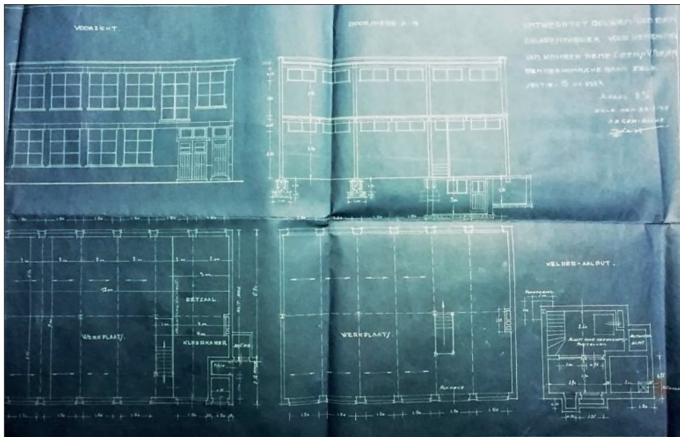
Plan van 1935 voor de sigarettenfabriek
